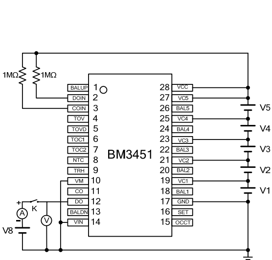
测试电路 7
