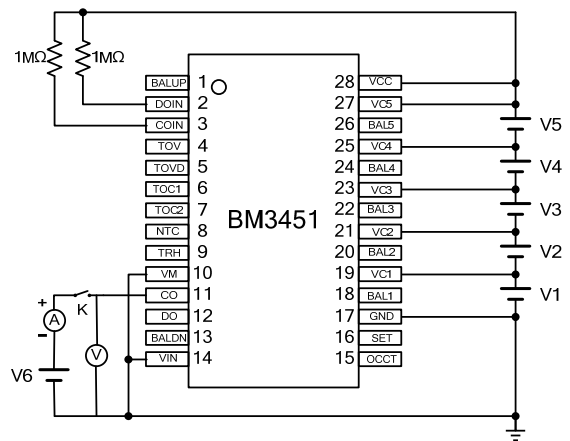
测试电路 6
