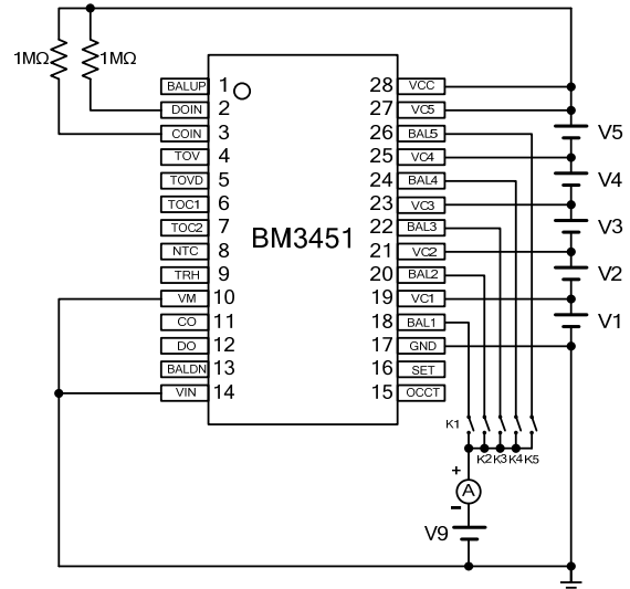
测试电路 8
