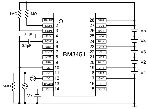
测试电路 4
